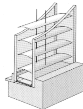
Figur 4. Opbygning af en 2-lags termorude med indbygget persienne.
