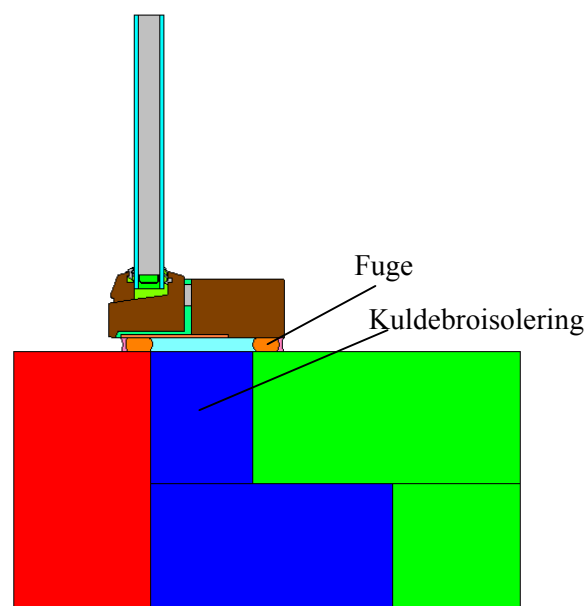
Figur 8. Placering af det smalle rammekarmprofil over kuldebroisoleringen.
