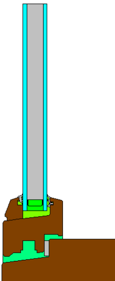
Figur 5, Trævinduet med smallere ramme og karm.
