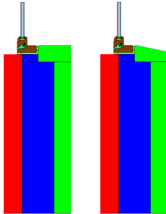
Figur 14. Ramme-karm af træ monteret i forskudt fals, hhv. retvinklet og skrå og med overkanten af falsen flugtende med karmen.
