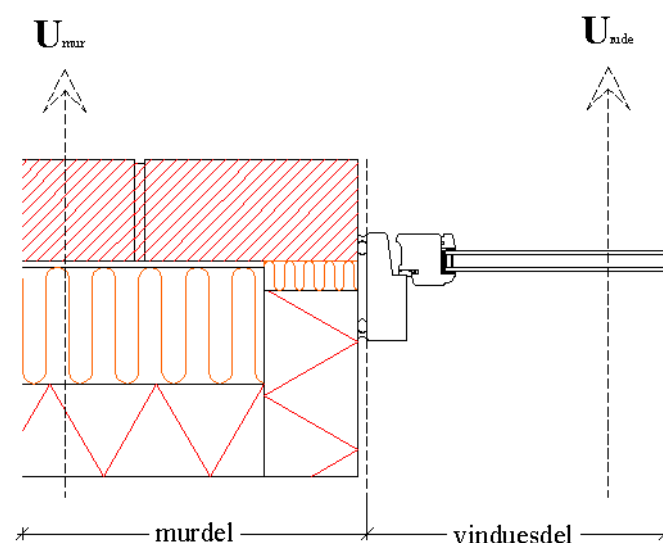
Figur 28. Længdeangivelse for beregning af de én-dimensionale varmetømme, \Phi_{1-dim} , gennem mur hhv. rude.
