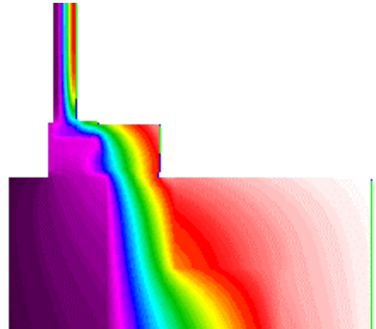
Figur 31. Ramme-karmkonstruktion af blandede materialer med murløsning med 190 mm isolering og 77 mm kuldebroisolering. Bemærk den store afbøjning af isothermerne fra rudens og ned til falsen
