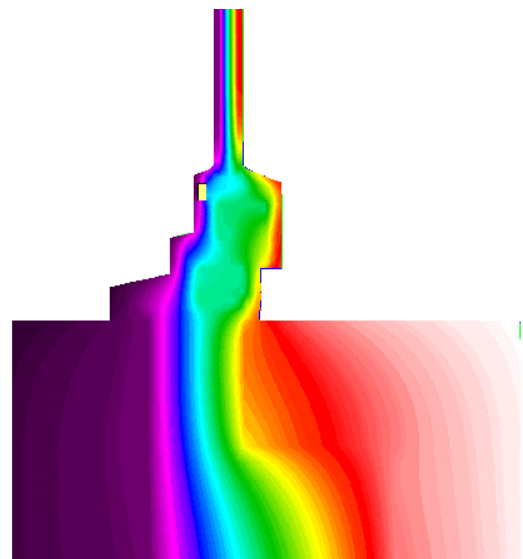
Figur 32. Ramme-karmkonstruktion af plast med murløsning med 190 mm isolering og 77 mm kuldebroisolering. Bemærk de forholdsvis rette isothermer i tilslutningen af karmen til falsen
