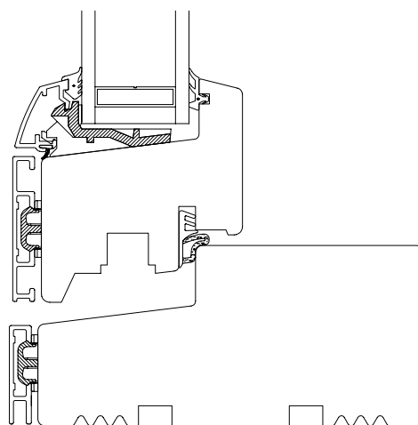
Figur 4. Bunden i ramme-karm af træ beklædt med aluminium (venstre side er udvendig side)
