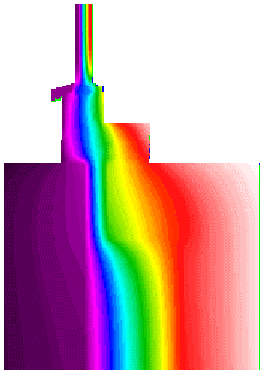
Figur 29. Isotermernes forløb ned gennem en mur-vinduekonstruktion med 125 mm isolering i mur og 32 mm isolering i kuldebro
