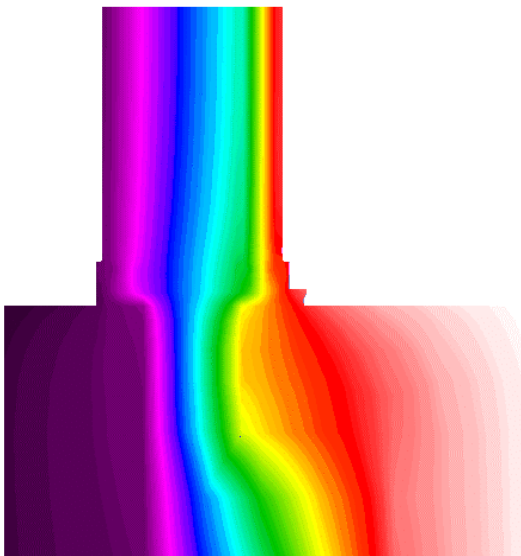
Figur 33. Kombinationsvinduet med murløsningen med 190 mm isolering og 77 mm kuldebroisolering. Bemærk indbøjningen af isothermerne ved tilslutningen til falsen
