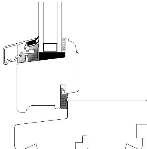
Figur 3. Bunden i ramme-karm af træ (venstre side er udvendig side)
