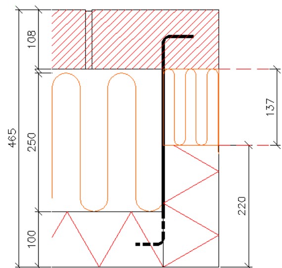
Figur 18. Murløsning med optimal isoleringstykkel på 250 mm og kuldebroisolering på 137 mm
