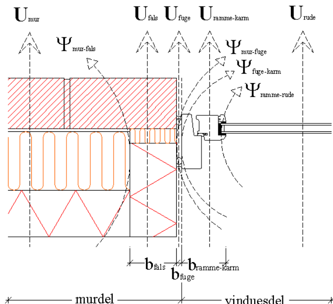
Figur 26. Bestanddelene i det udvidede linjetab, L
